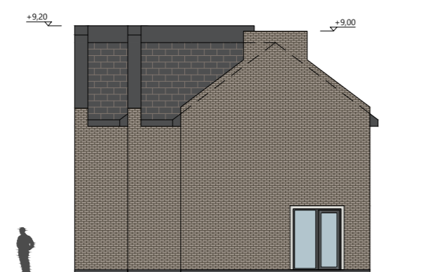
RYTINIS FASADAS
