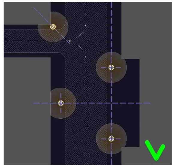
Pav.4.6. Šviestuvų dėstymo rekomendacijos. 1 – mechanišku dėstymo ritmu neardyti erdvių kompozicijos; 2 - atsižvelgti į konkrečią erdvės specifiką (išnaudoti gatvių kampus, pabrėžti vertingus erdvių elementus);
