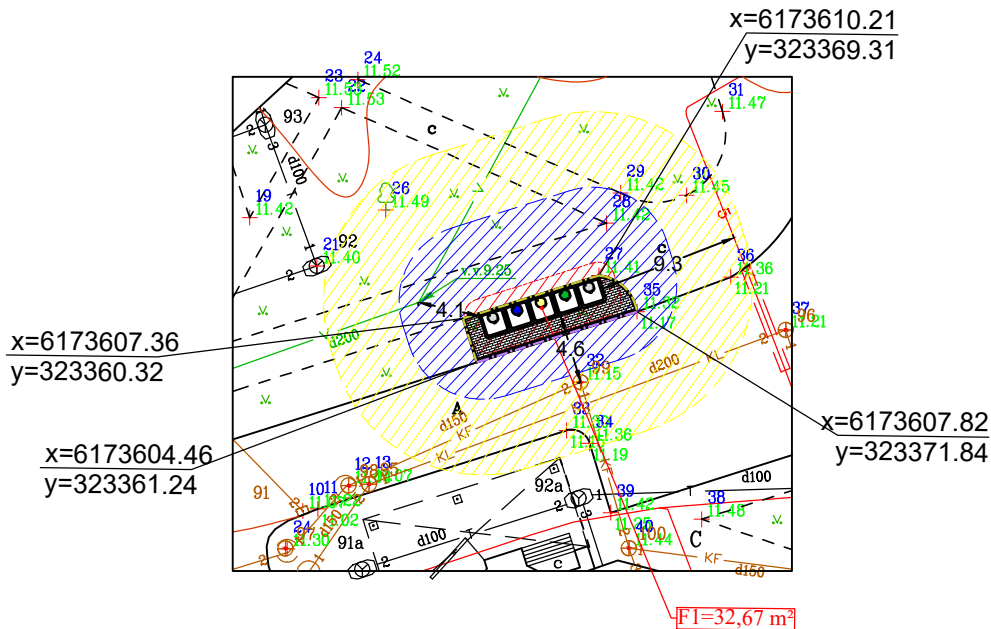
PUSIAU POŽEMINIŲ KONTEINERIŲ AIKŠTELĖS ĮRENGIMO SCHEMA M 1:500
