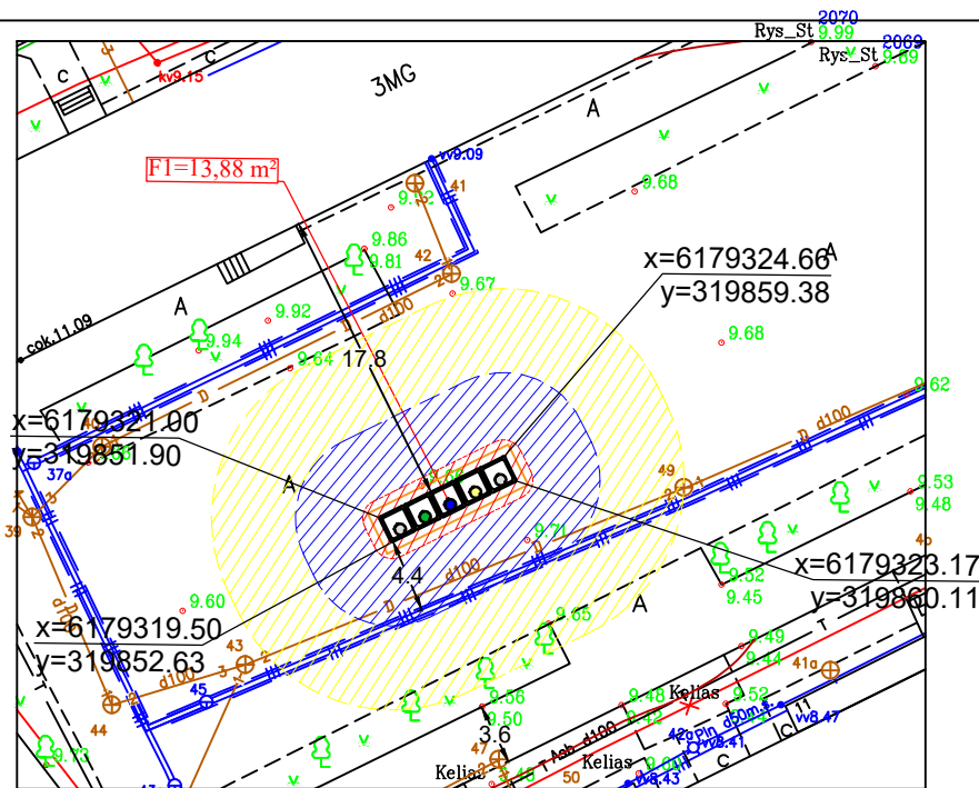
PUSIAU POŽEMINIŲ KONTEINERIŲ AIKŠTELĖS ĮRENGIMO SCHEMA M 1:500
