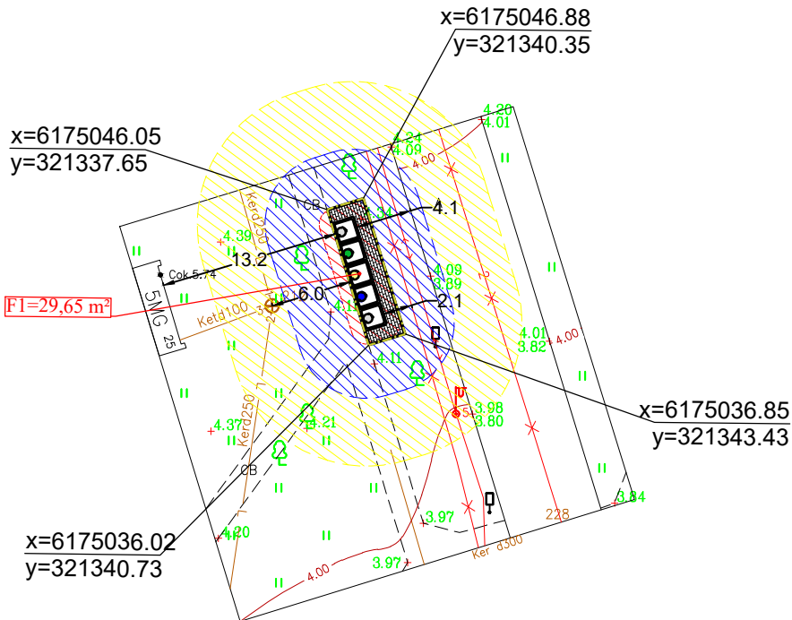
PUSIAU POŽEMINIŲ KONTEINERIŲ AIKŠTELĖS ĮRENGIMO SCHEMA M 1:500
