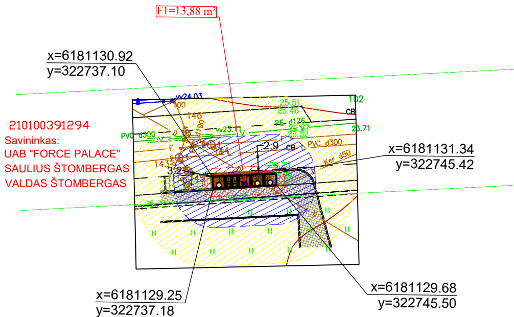
PUSIAU POŽEMINIŲ KONTEINERIŲ AIKŠTELĖS ĮRENGIMO SCHEMA M 1:500
