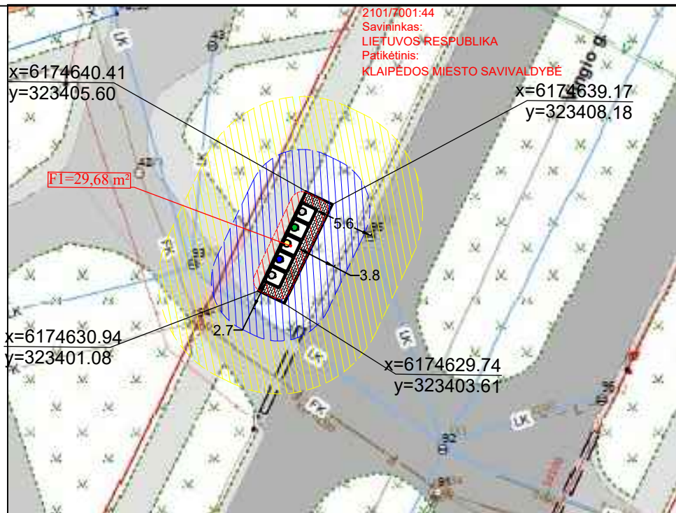
PUSIAU POŽEMINIŲ KONTEINERIŲ AIKŠTELĖS ĮRENGIMO SCHEMA M 1:500
