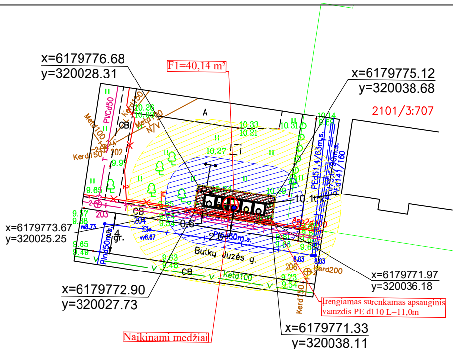
PUSIAU POŽEMINIŲ KONTEINERIŲ AIKŠTELĖS ĮRENGIMO SCHEMA M 1:500
