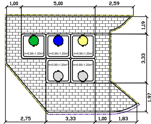
BUITINIŲ ATLIEKŲ PUSIAU POŽEMINIŲ KONTEINERIŲ AIKŠTELĖ
