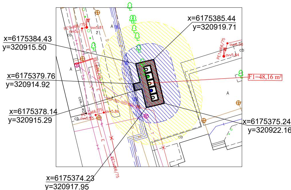
PUSIAU POŽEMINIŲ KONTEINERIŲ AIKŠTELĖS ĮRENGIMO SCHEMA M 1:500
