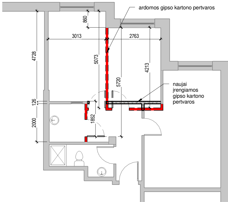
ARDYMO DARBŲ PLANAS, m 1:100
