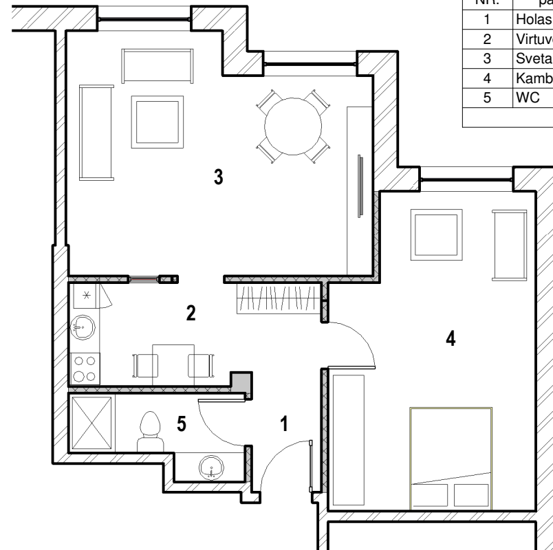
PATALPŲ PLANAS PO PERPLANAVIMO, m 1:100
