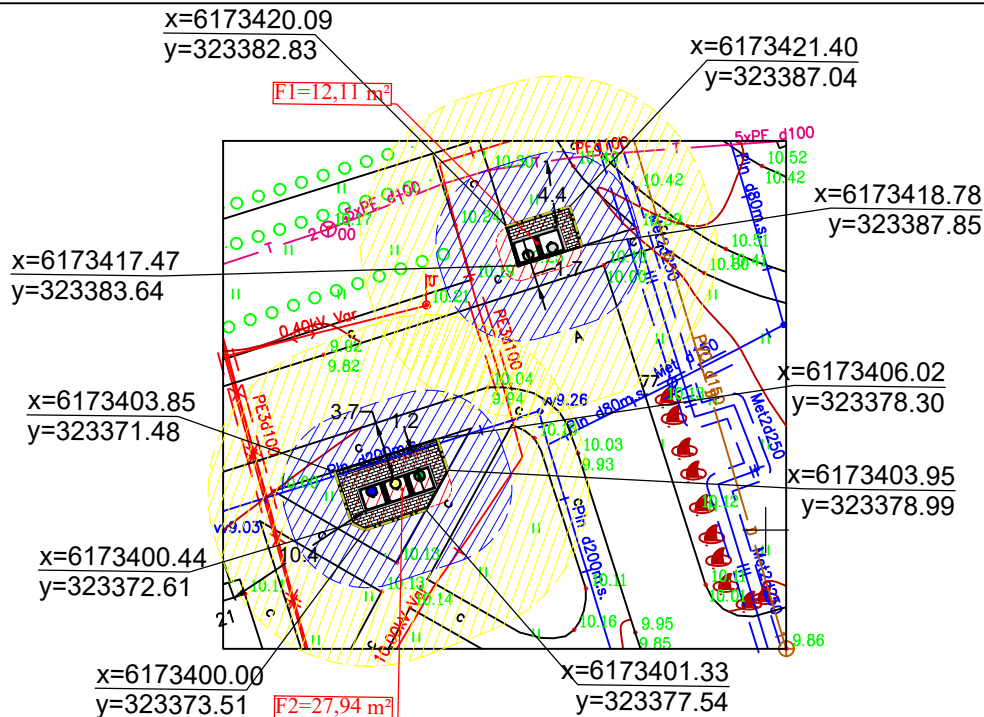
PUSIAU POŽEMINIŲ KONTEINERIŲ AIKŠTELĖS ĮRENGIMO SCHEMA M 1:500
