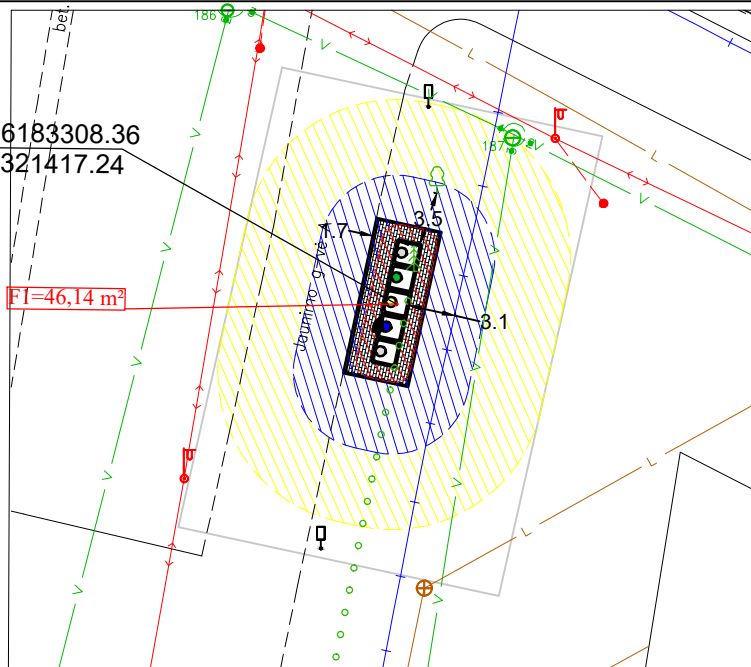
PUSIAU POŽEMINIŲ KONTEINERIŲ AIKŠTELĖS ĮRENGIMO SCHEMA M 1:500
