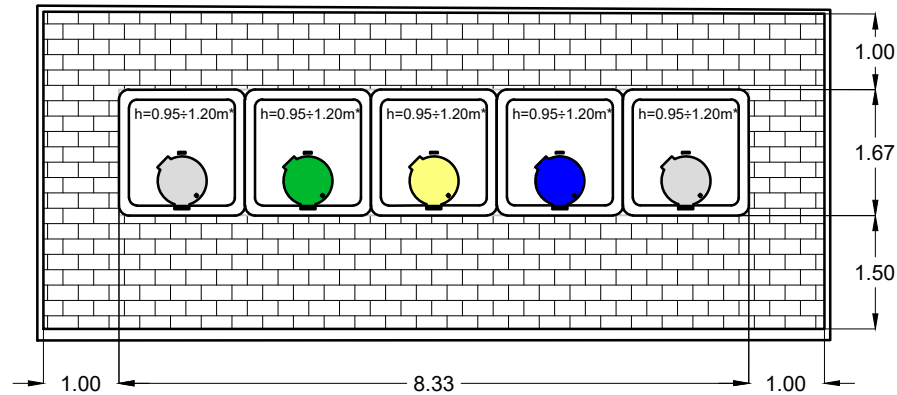
BUITINIŲ ATLIEKŲ PUSIAU POŽEMINIŲ KONTEINERIŲ AIKŠTELĖ
