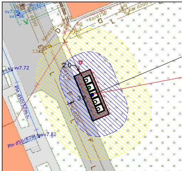
PUSIAU POŽEMINIŲ KONTEINERIŲ AIKŠTELĖS ĮRENGIMO SCHEMA M 1:500
