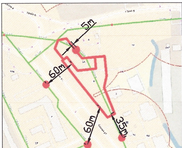
Hidrantų schema
