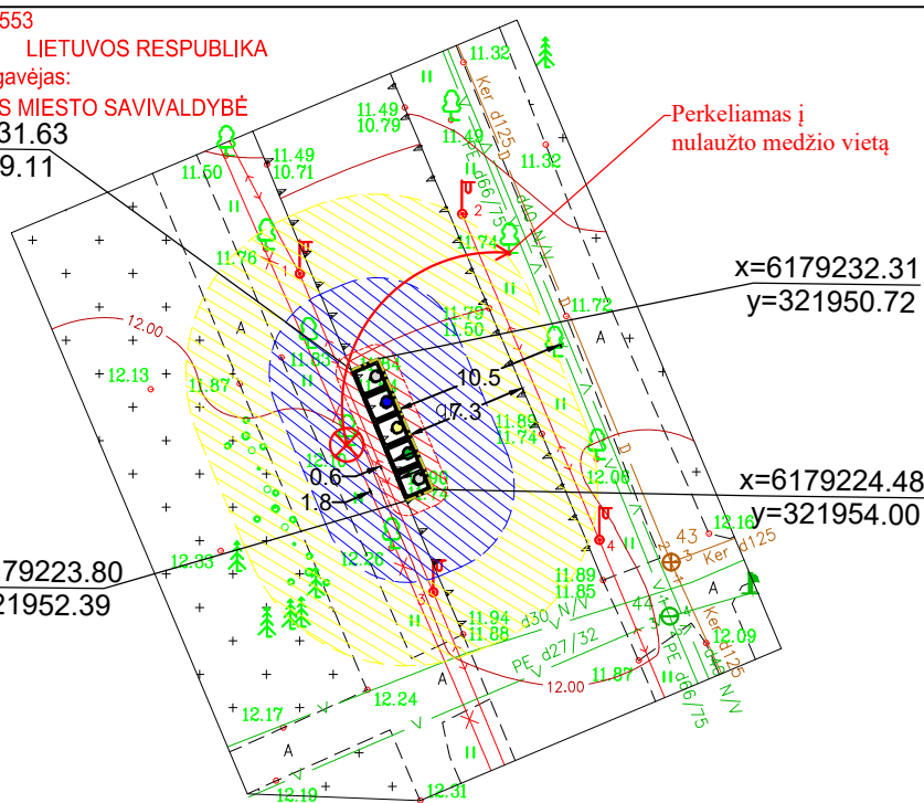
PUSIAU POŽEMINIŲ KONTEINERIŲ AIKŠTELĖS ĮRENGIMO SCHEMA M 1:500
