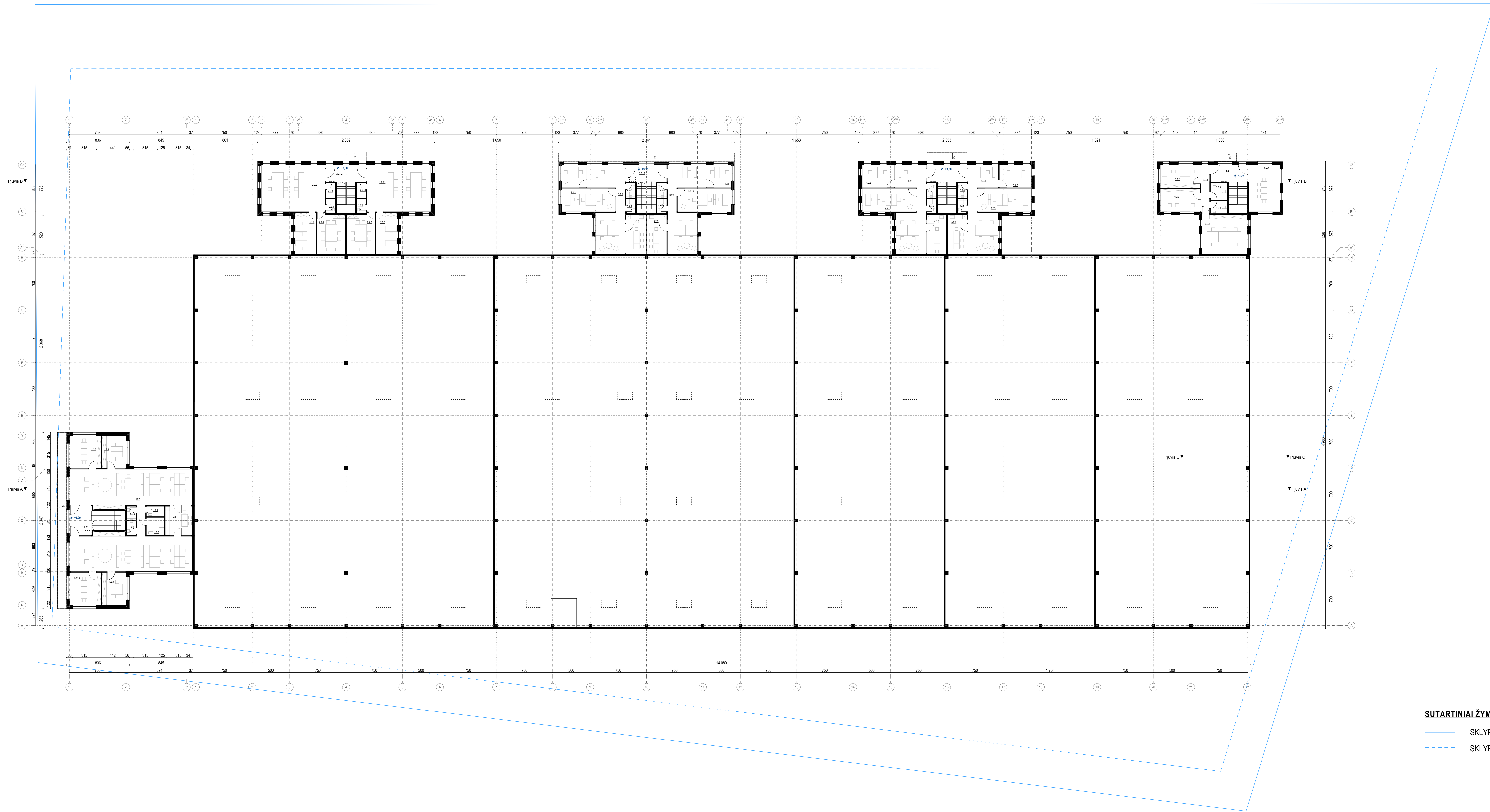
Šešių blokuotų gamybos paskirties pastatų dalinimo schema
