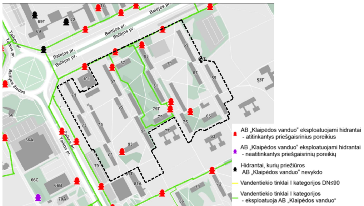
2.12.1. Esamų gaisrinių hidrantų išdėstymo schema.
