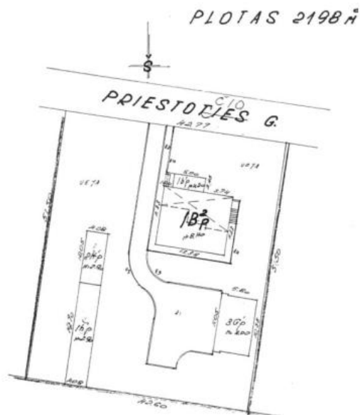
1979 m. statinių išdėstymo planas
