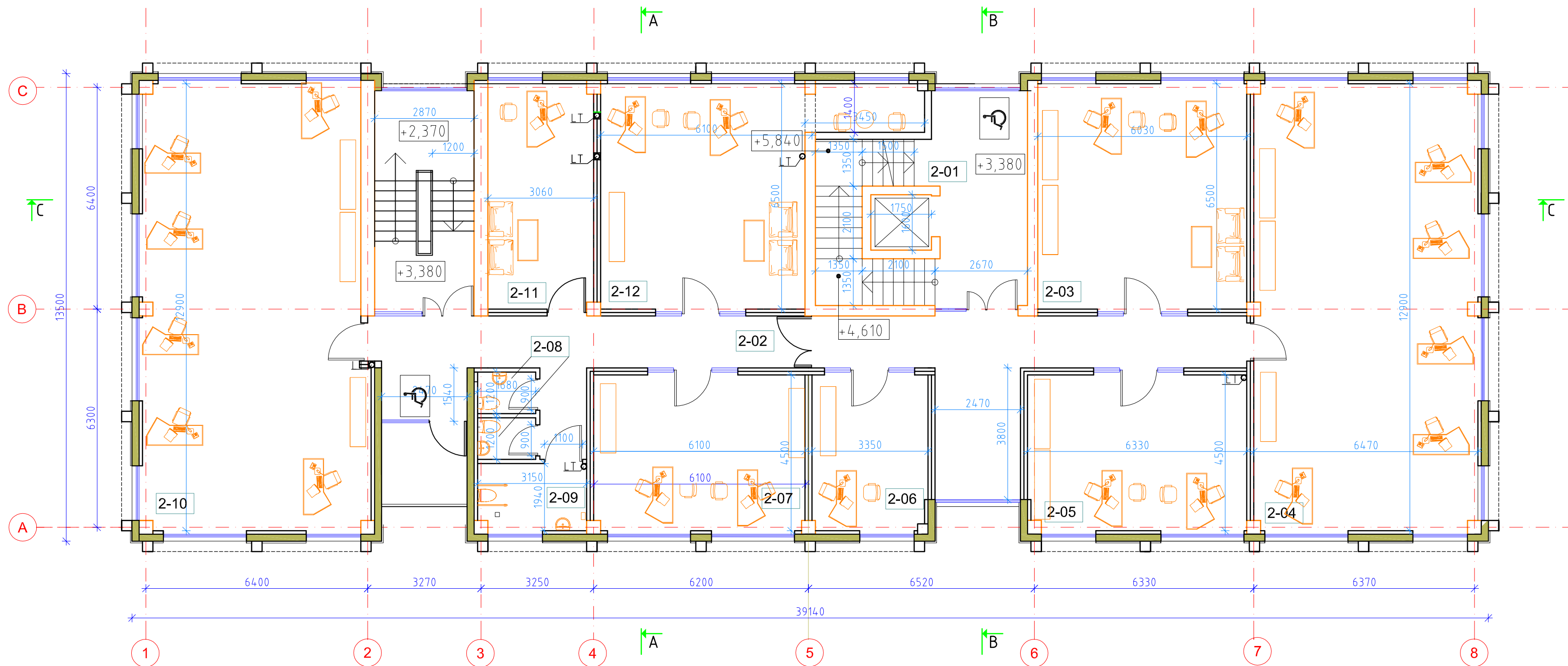
PATALPŲ EKSPLIKACIJA
