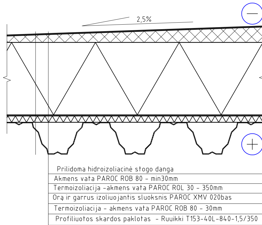
STOGO DETALĖ ST2 U=0,092W/m^2K
