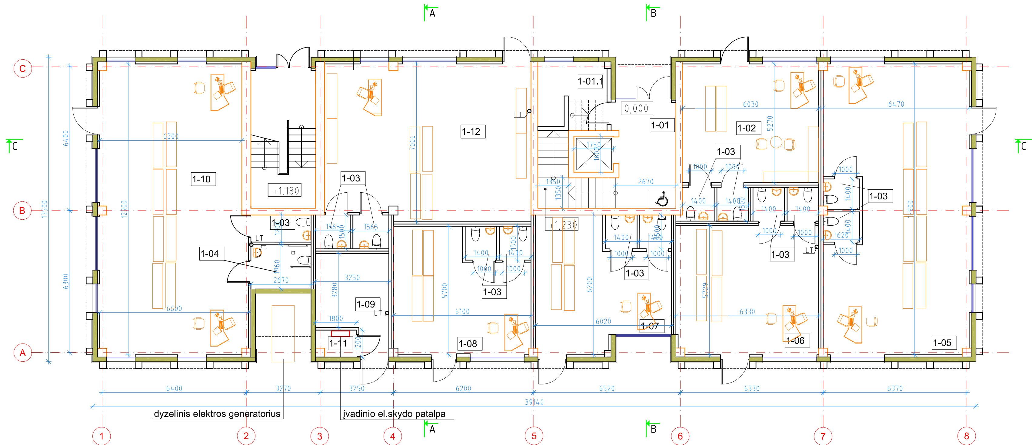
PATALPŲ EKSPLIKACIJA
