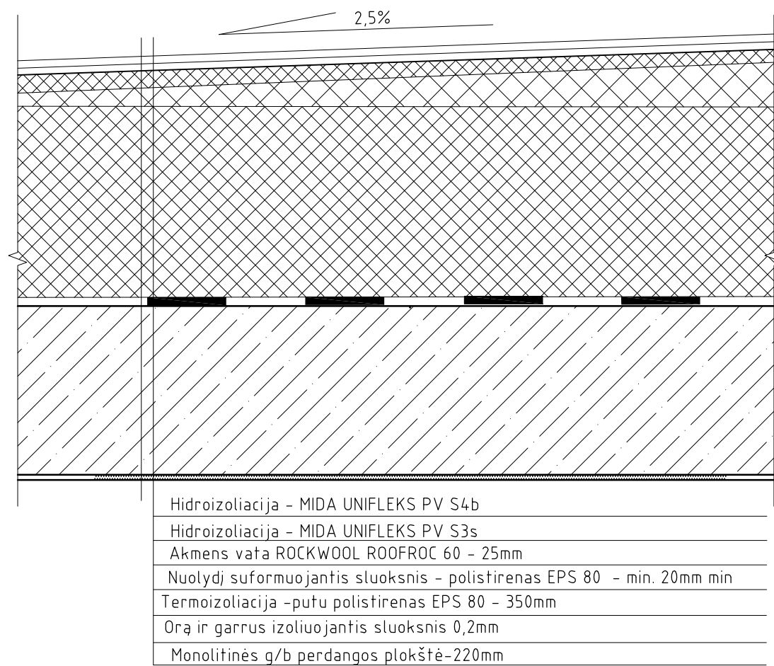
STOGO DETALĖ ST1 U=0,097W/m^2K
