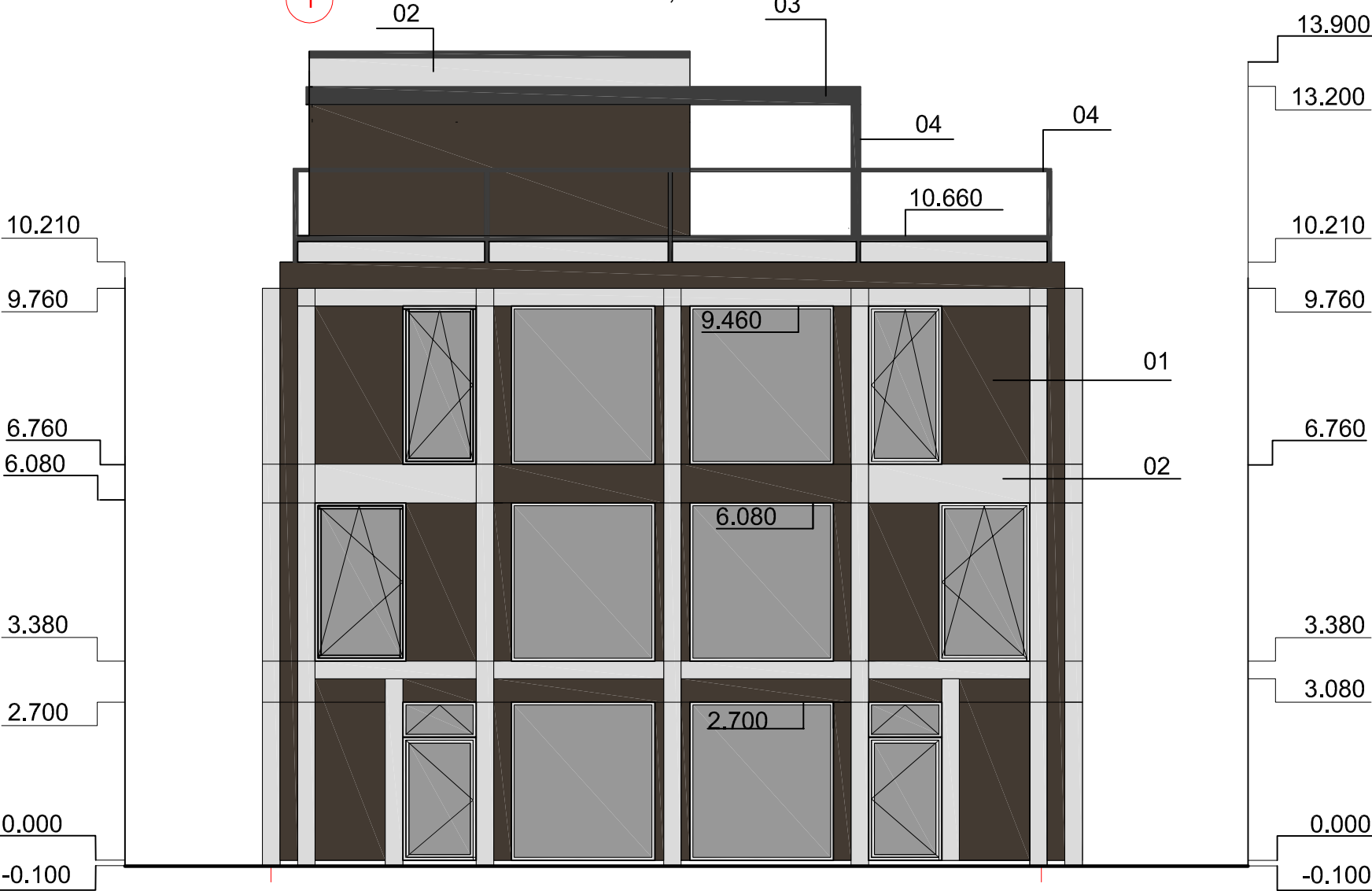
FASADAS C-A, M1:100
